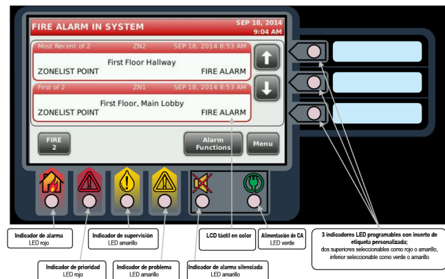
Figura 2: Pantalla táctil con indicadores LED de estado
